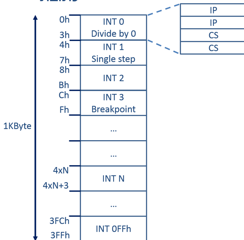
מבנה ה-Interrupt Vector Table בזיכרון
